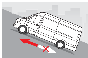
Asistent pro rozjezd do kopce HAC (Hill Assist Control)
