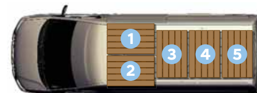
Dlouhý rozvor (5 europalet)
